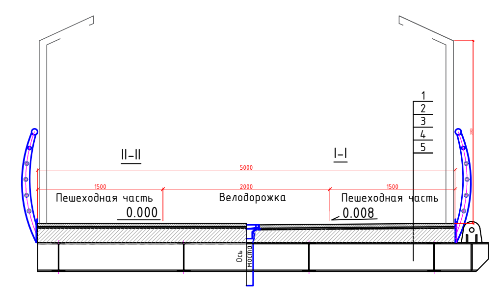
Сечение моста
